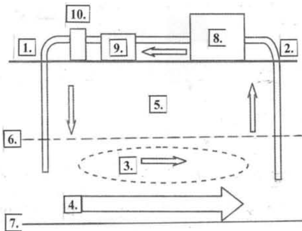
Slika 5. Šematski prikaz bipolarnog modela [2] Fig. 5 Schematic preview of bipolar model [2]
