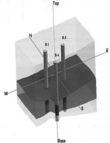
Slika 6. 3D prikaz bipolarnog modela za bioremedijaciju podzemnih voda na lokaciji L2 Fig. 6 3D preview of bipolar model for bioremediation of groundwater at the site L2
