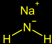
NATRIJUM AMID
