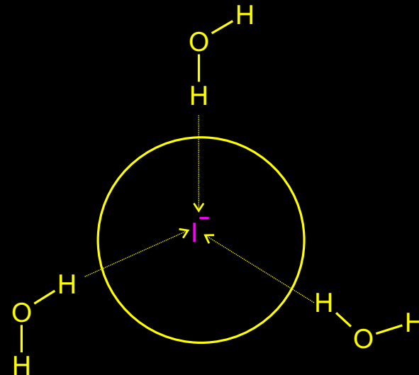
SLABA SOLVATACIJA I - ANJONA
