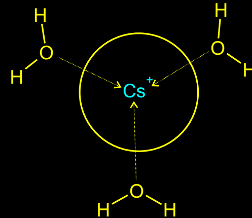
SLABA SOLVATACIJA Cs + KATJONA
