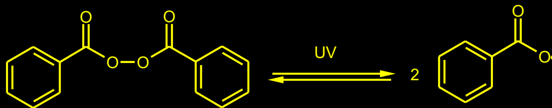
BENZOILPEROKSID
