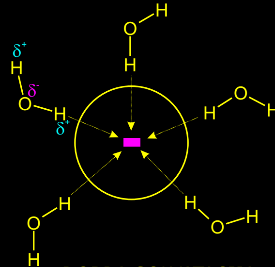
DOBRA SOLVATACIJA
